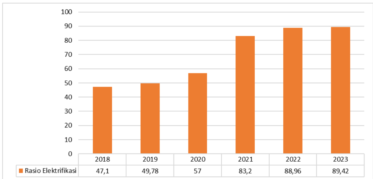
Gambar 2.64. Grafik Rasio Elektrifikasi Kabupaten Seruyan Tahun 2018-2023
